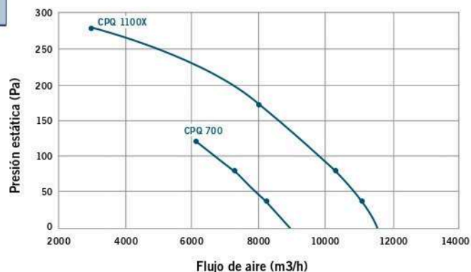
CURVA DEL VENTILADOR
